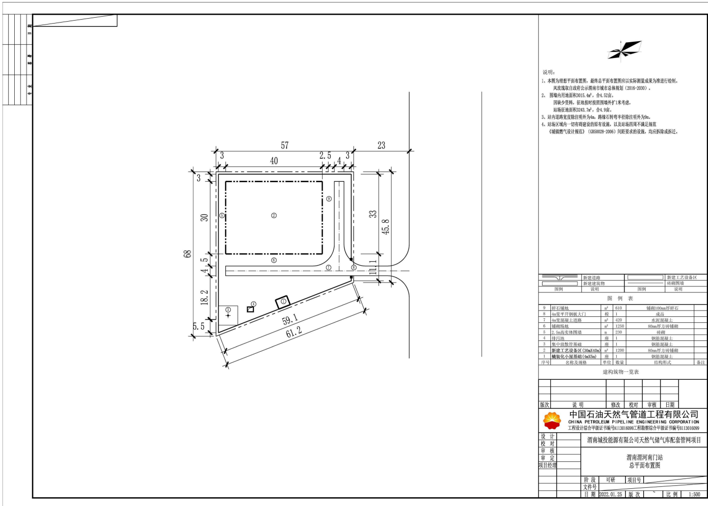
附图6 南门站平面布置图
