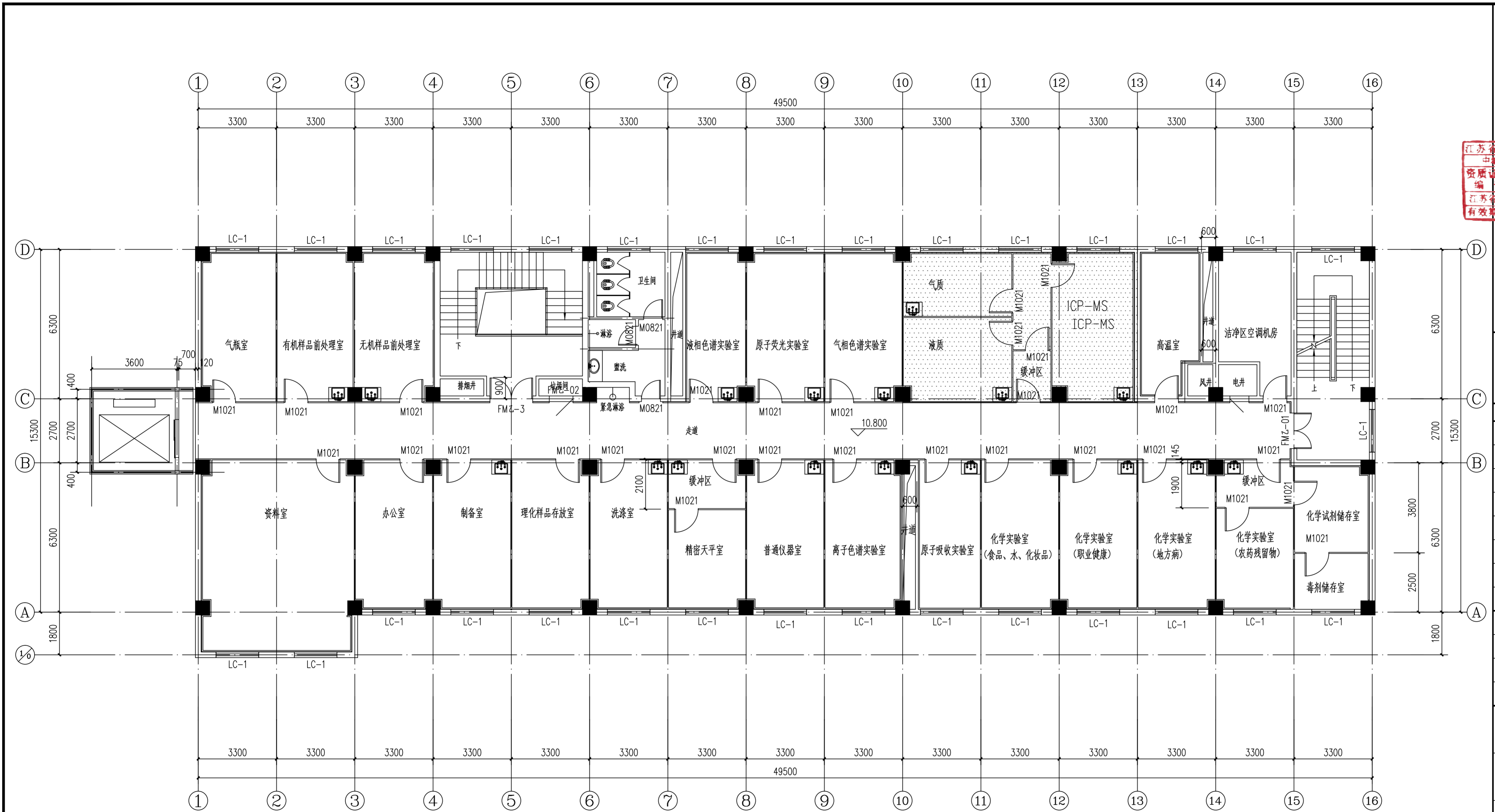
四层改造平面图 1:100
