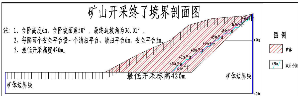
图 1.3-2 开采终了剖面图
