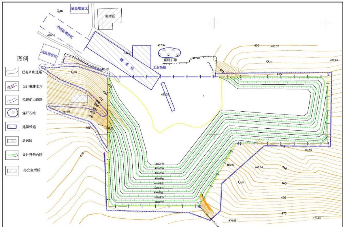
图 1.3-3 矿山工程平面布置示意图
