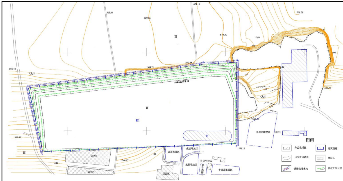
图 1.3-3 矿山工程平面布置示意图
