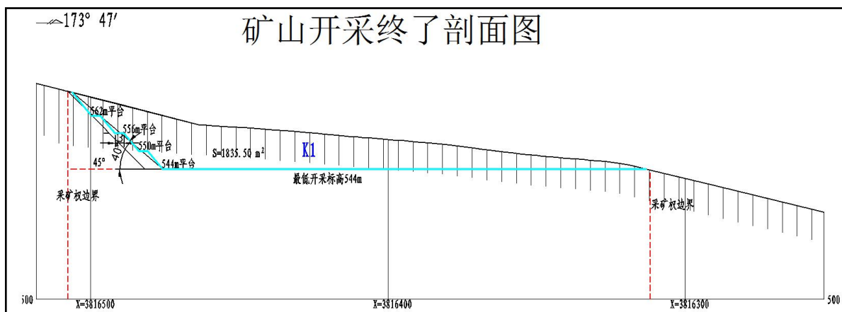
图 1.3-2 开采终了剖面图
