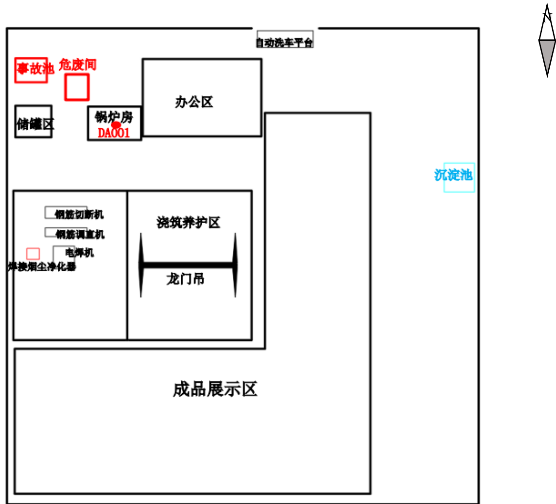
附图 3 项目总平面布置图
