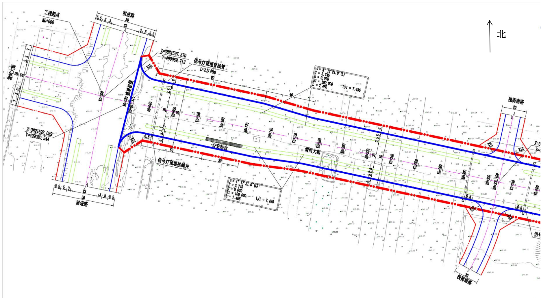
附图 5-1: 平面布置图 (前进路--槐街南路段)
