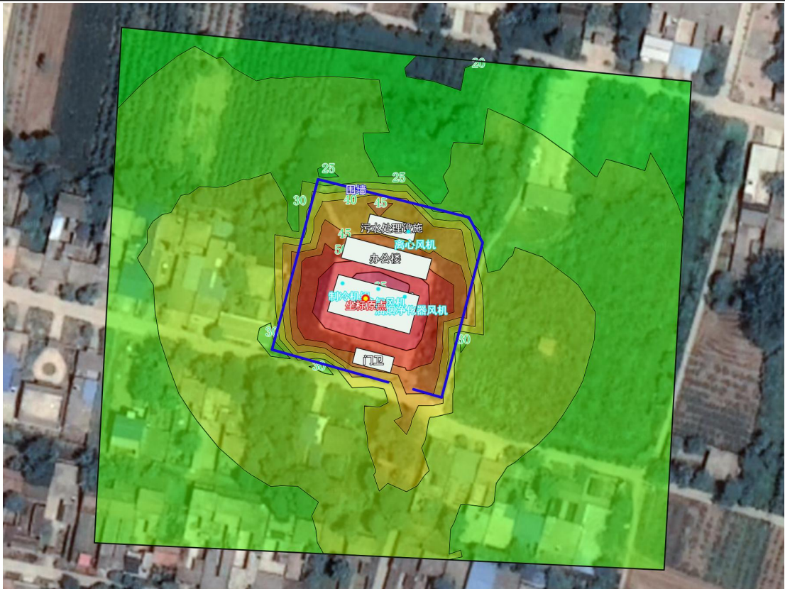
图 4-4 项目昼间噪声等值线图
