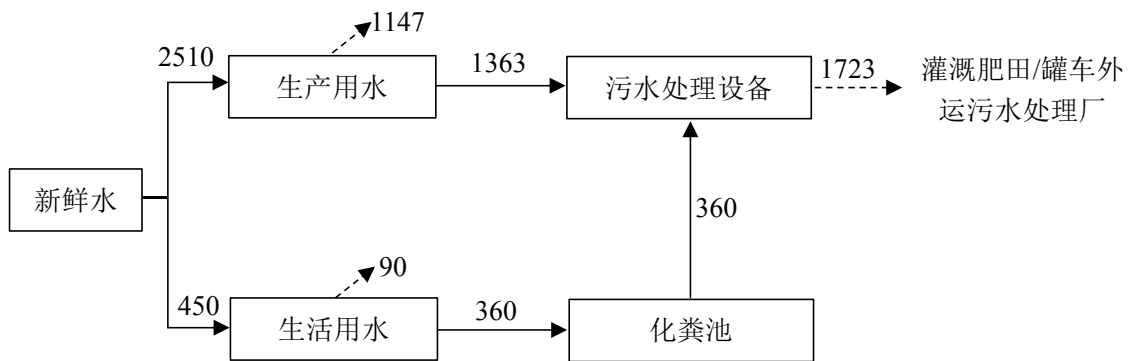
图 4-1 运营期用水量平衡图 单位：m 3 /a
