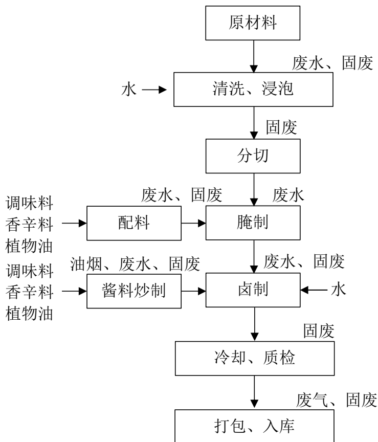
图 2-3 酱卤副产品生产工艺及产污环节图
