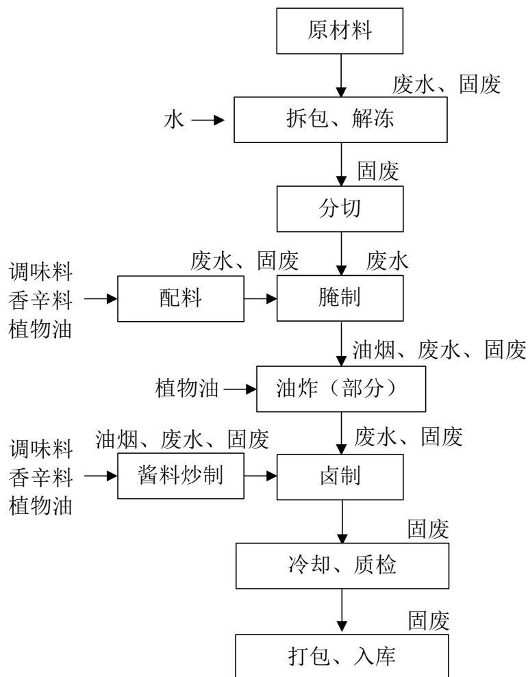
图 2-4 酱卤肉制品生产工艺及产污环节图
