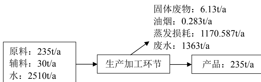
图 2-1 物料平衡图
